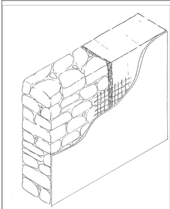
Figure 22: Joint droit et enduit
