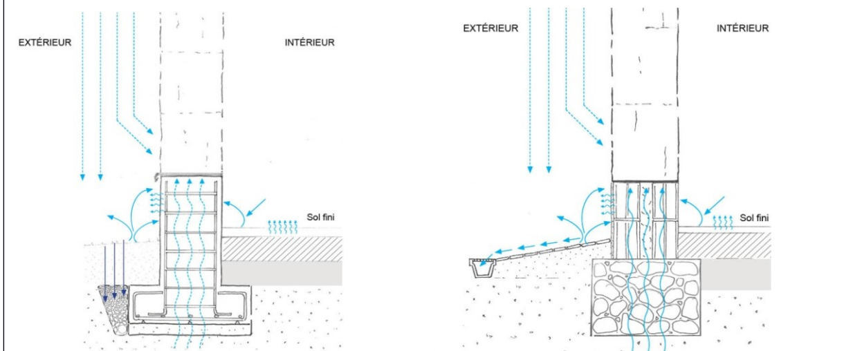
Figure 14: Fondation pierres, soubassement* isolant, sol en pierre, canal drainant
