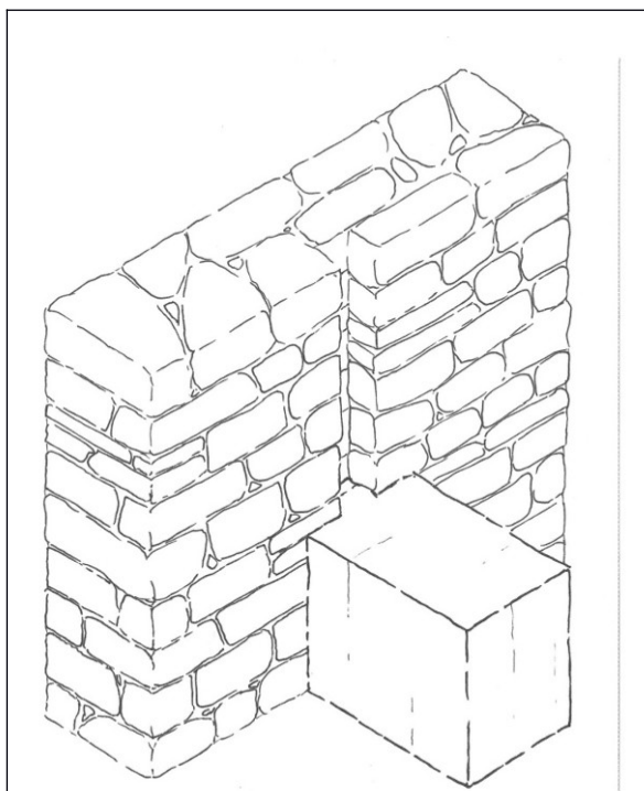
Figure 20: Mur en pierre avec saignées* de 5×5 cm ou 10×10 cm dans lequel le mur vient rentrer.
